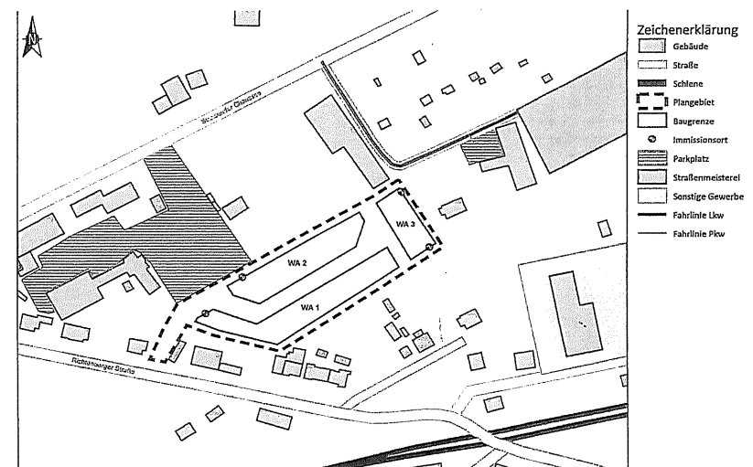
Abbildung 4-1 Übersicht der Anlagenschallquellen
