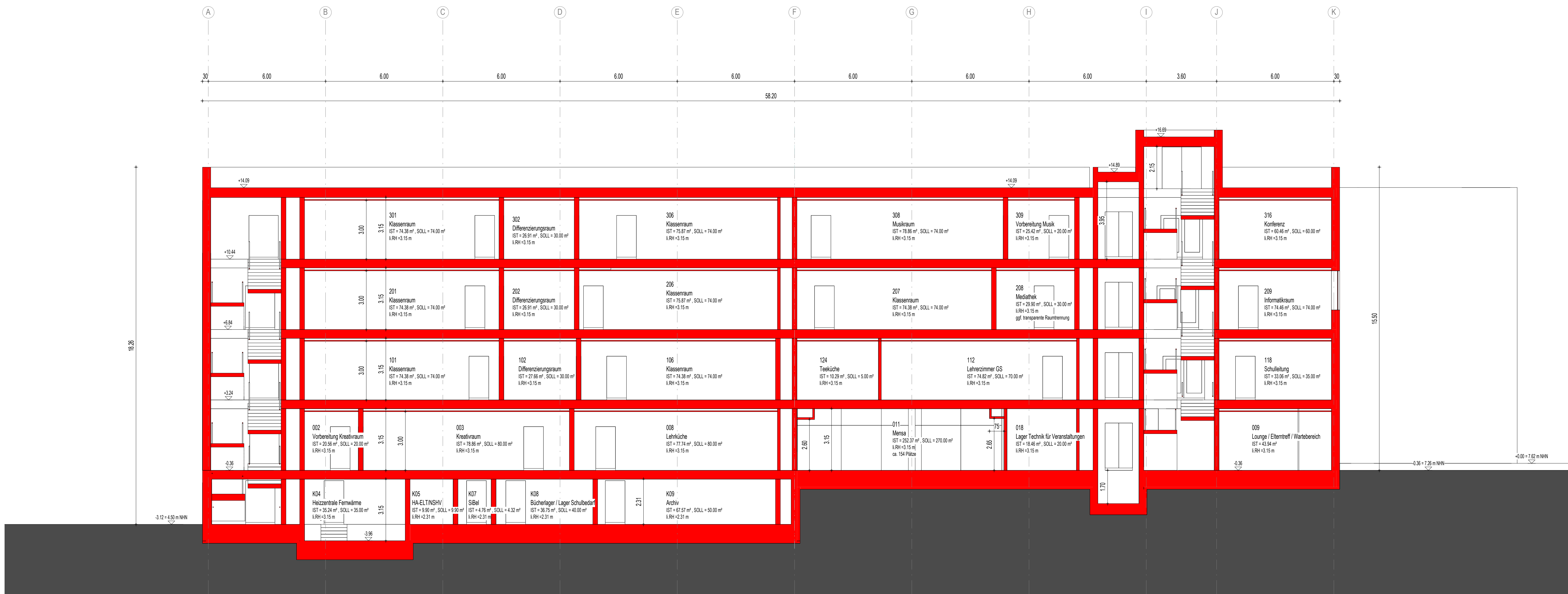
Längsschnitt
