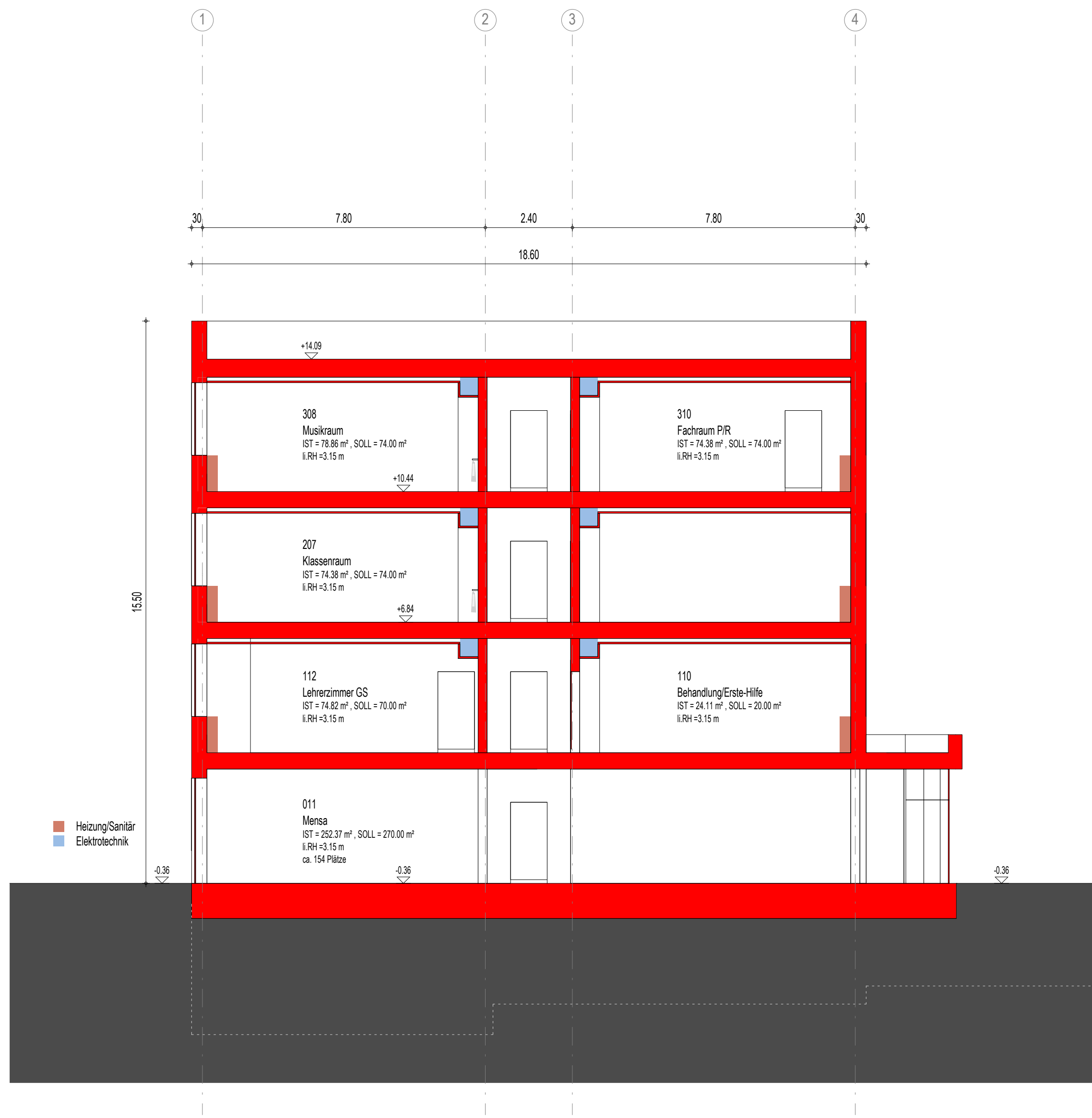
Querschnitt
