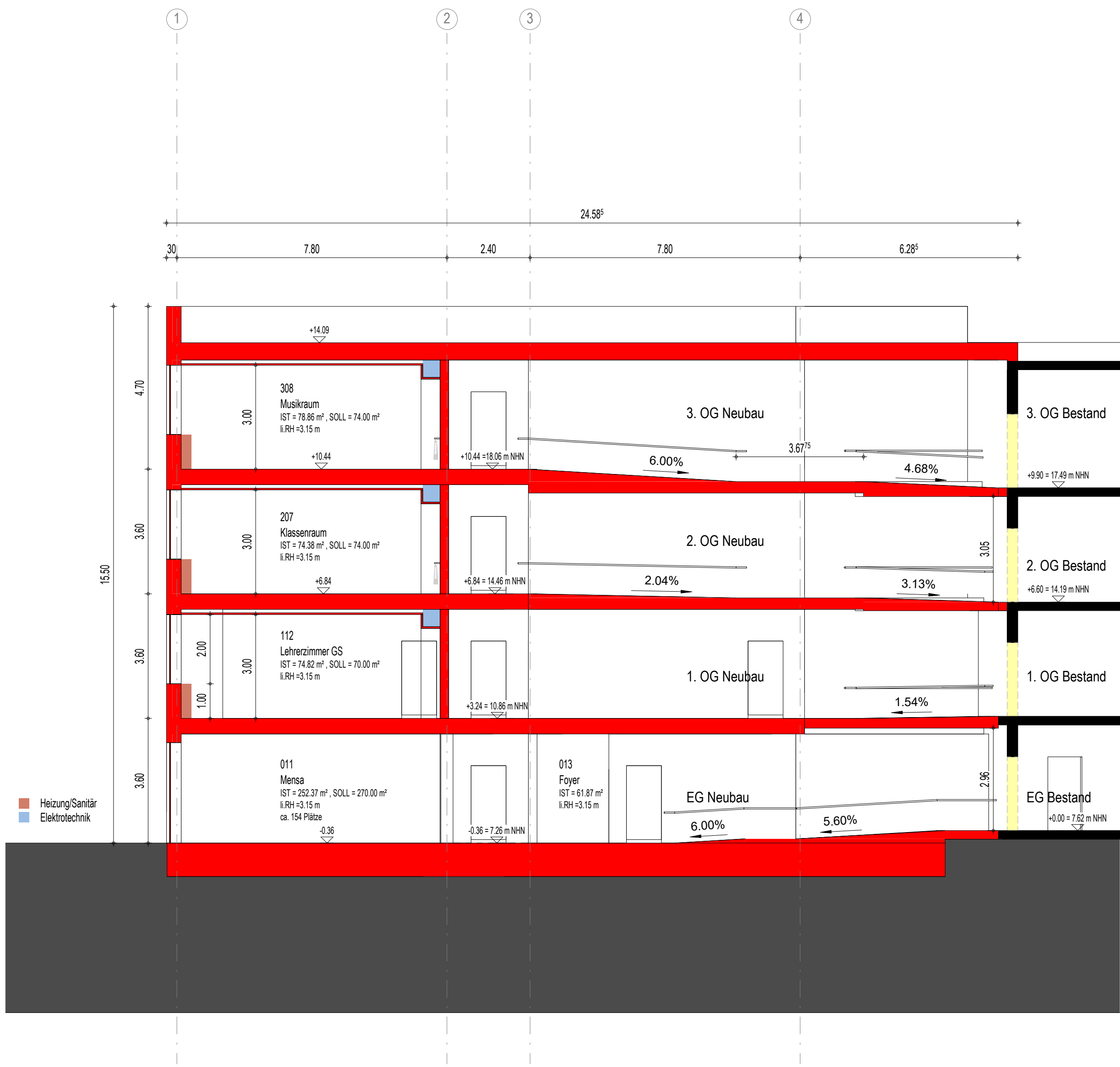
Querschnitt Rampe
