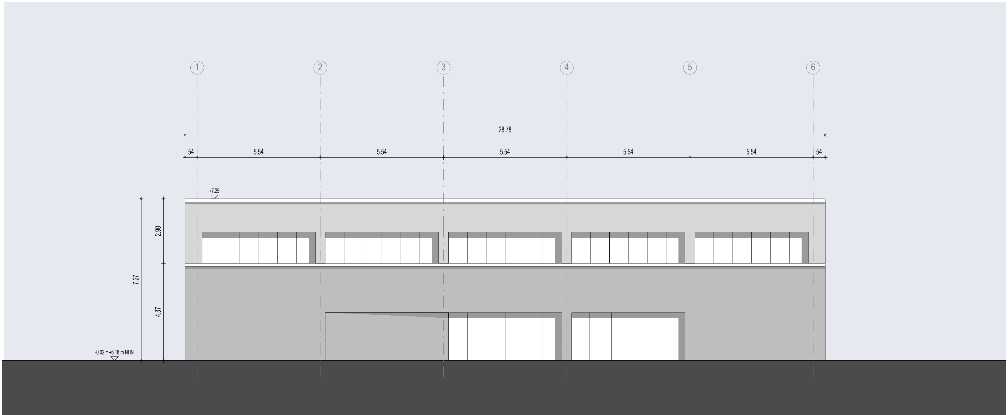
Fassade Ansicht Süd
