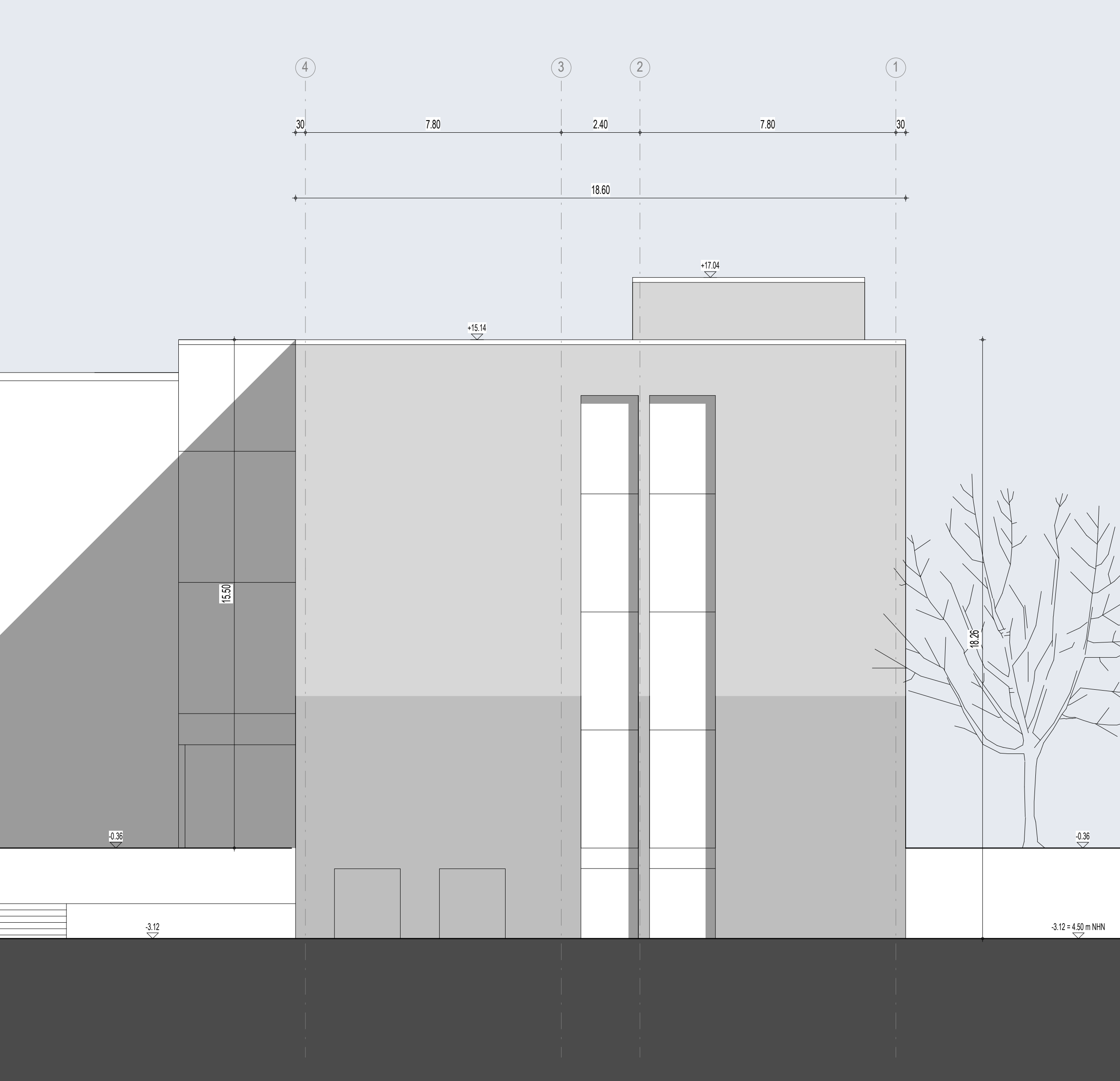
Fassade Ansicht Nord
